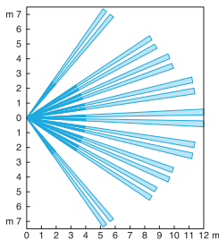
Erfassungsbereich Draufsicht LX-402
